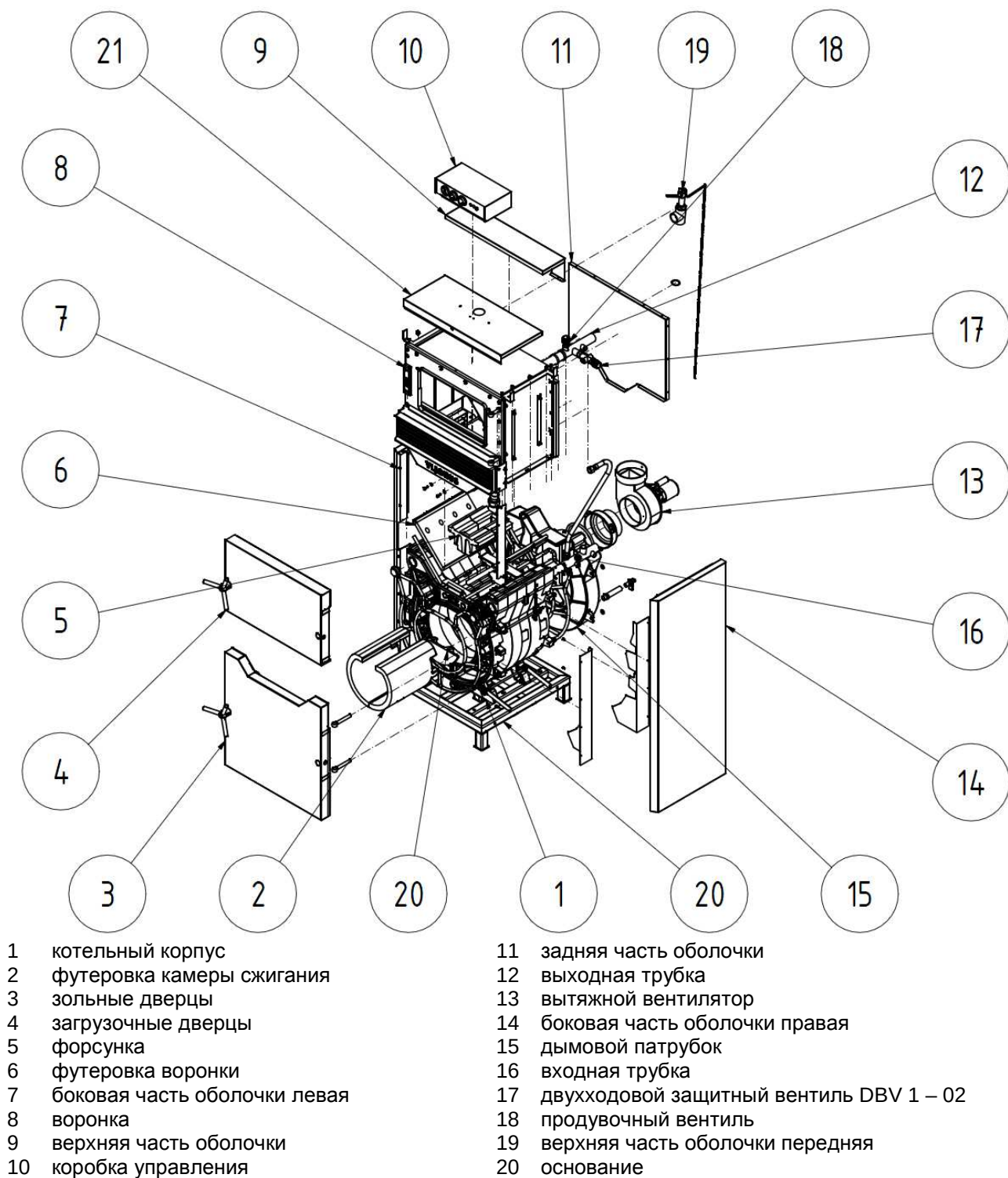
Рис.. 4b) Главные части котла Hefaistos P1 E
