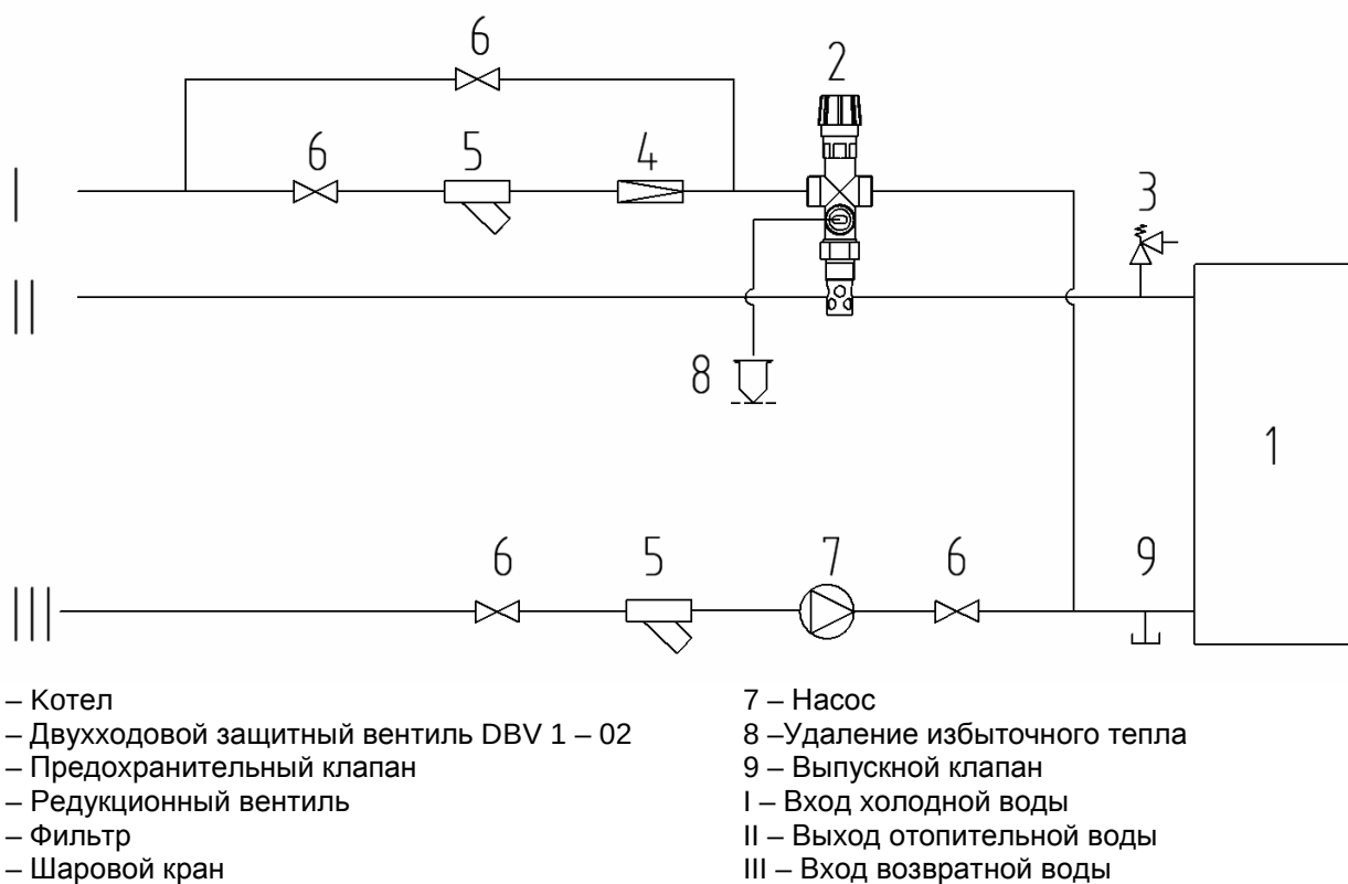
Рис. 15 Рекомендуемая схема включения двухходового защитного вентиля DBV 1 - 02
