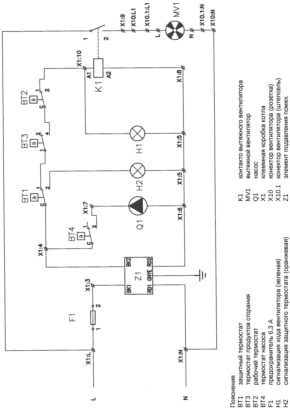
Рис. 19 Контурная схема включения котла Hefaistos P1 T
