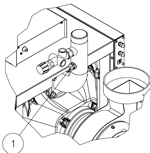
Рис. № 15 Размещение гильзы датчика ОВ
