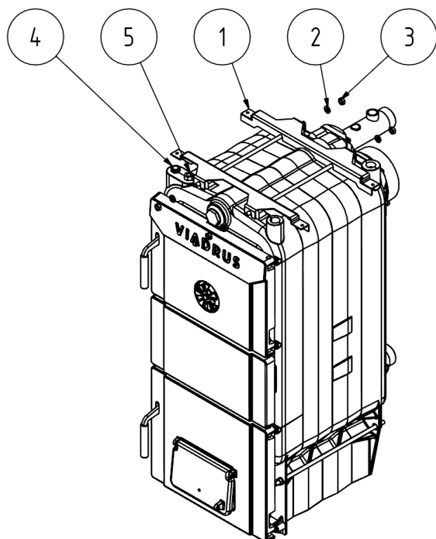
Рис. № 13 Монтаж консолей оболочки
