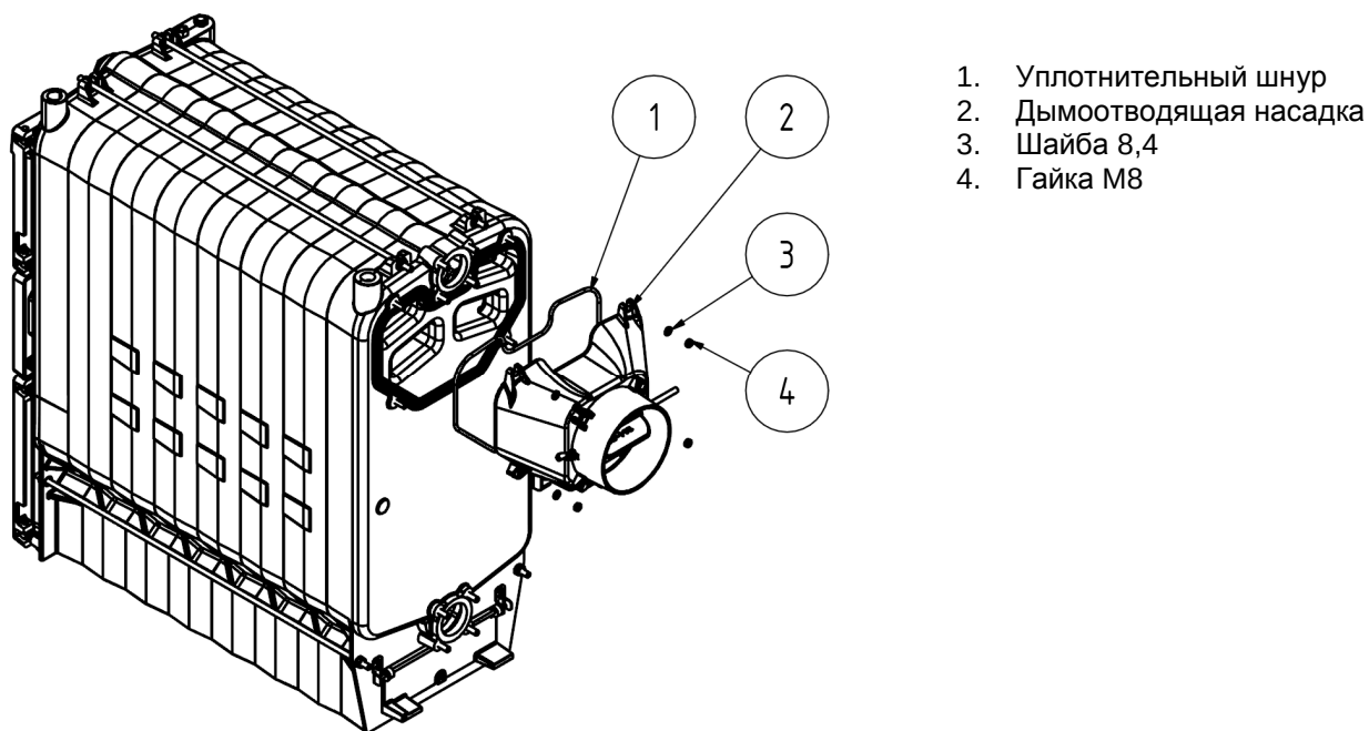
Рис. № 11 Установка дымоотводящей насадки
