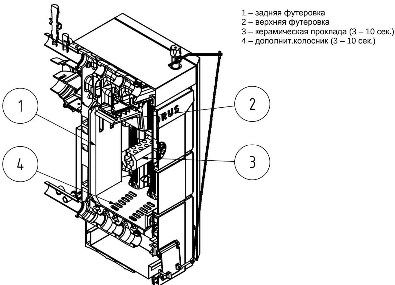
Рис. № 4с) Схема котла VIADRUS HERCULES U 26 – расположение дополнит.оснащения
