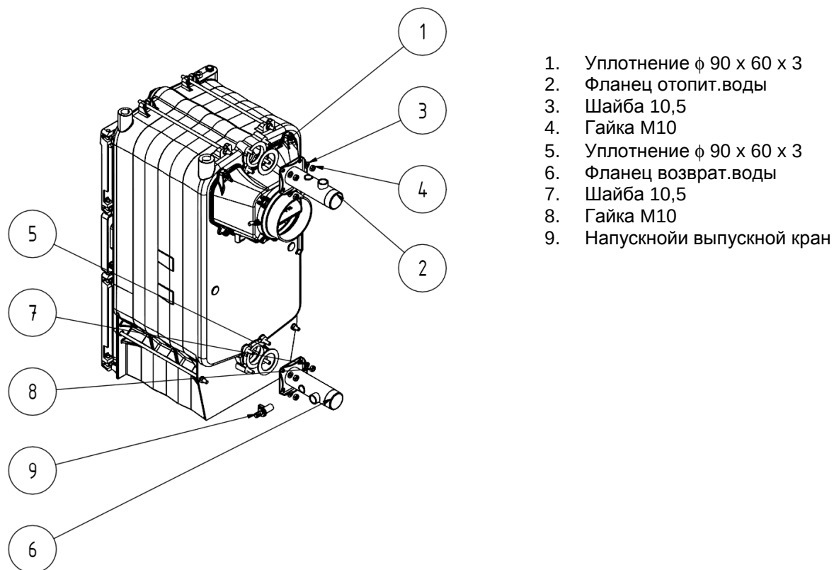
Рис. № 12 Установка котельного корпуса
