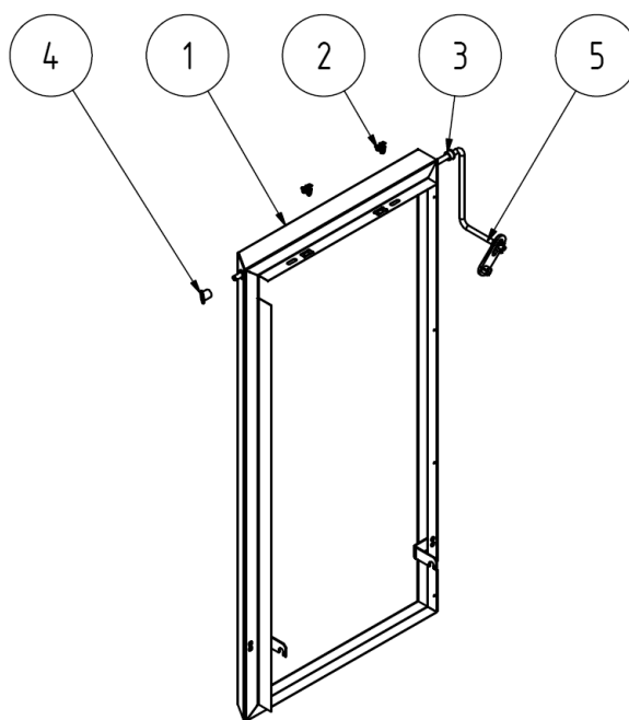
Рис. № 13 Монтаж консолей оболочки
